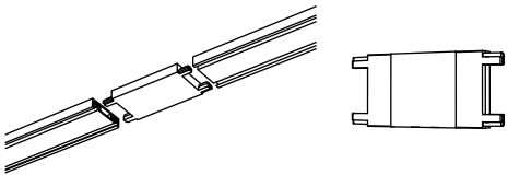
1. "Passagem": trilho diretamente emendado e eletrificado
